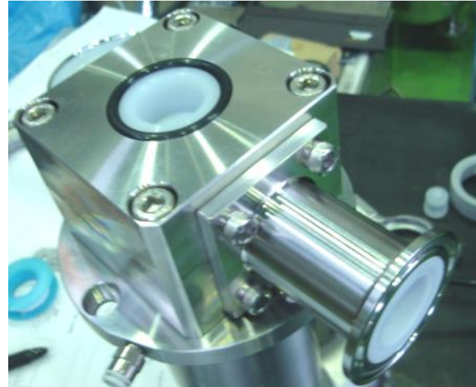
ALL-PTFE コネクタ外観
